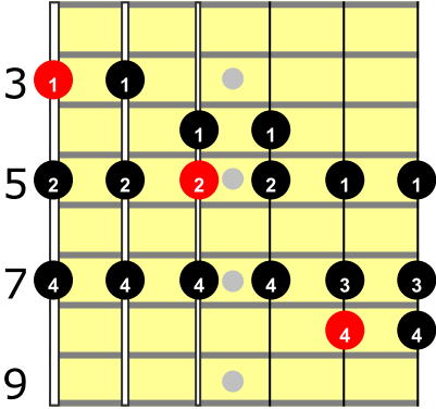
G IONIAN
