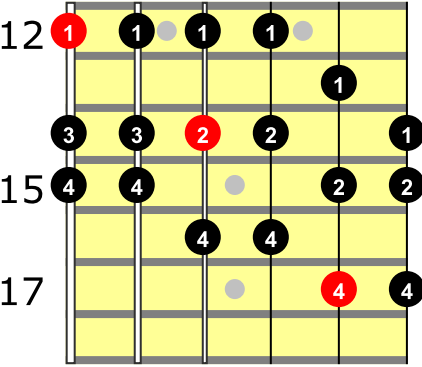
E AOLIAN
