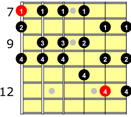
B PHRYGIAN
